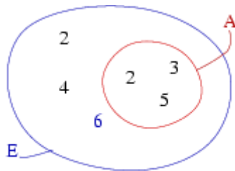
Sous-ensemble A d'un ensemble E
